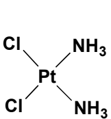
cisplatin
