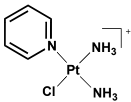
pyriplatin
