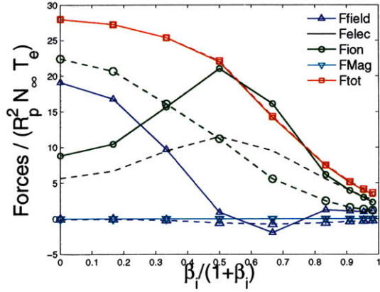
(d) e_x -axis
