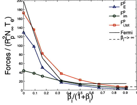
(d) \tau = 0.1, v_d = c_{s0}, \lambda_{De} = 30
