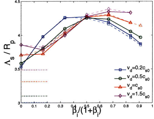
(d) \tau = 0.1, \lambda_{De} = 1
