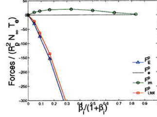
(l) v_d = 1.5c_{s0} , \lambda_{De} = 20
