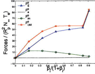
(h) v_d = c_{s0} , \lambda_{De} = 3
