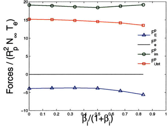
(d) v_d = c_{s0} , \mathbf{e}_x -axis
