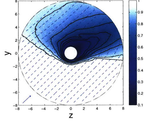
(d) \lambda_{De} = 1
