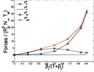
(d) v_d = 0.5c_{s0} , \lambda_{De} = 0.3
