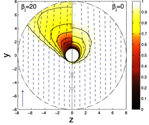
(d) \tau = 0.1, v_d = 0.5c_{s0}, \delta = \pi/8
