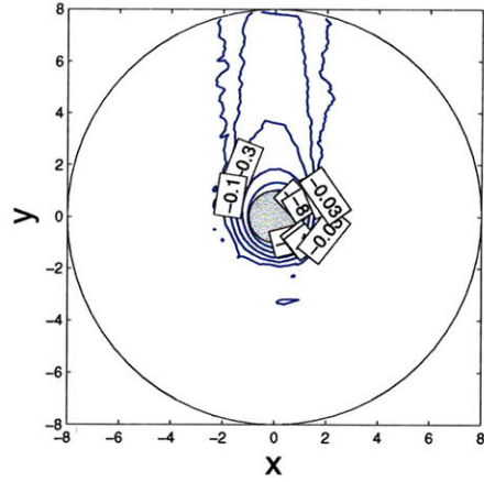
(d) \{0, \mathbf{e}_x, \mathbf{e}_y\} , \lambda_{De} = 3
