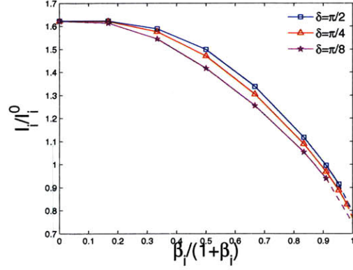
(d) \tau = 1, v_d = 1.5c_{s0}
