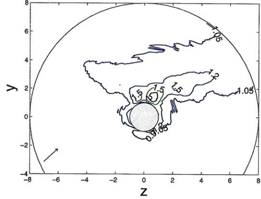
(d) T_{i,yy}, \lambda_{De} = 3
