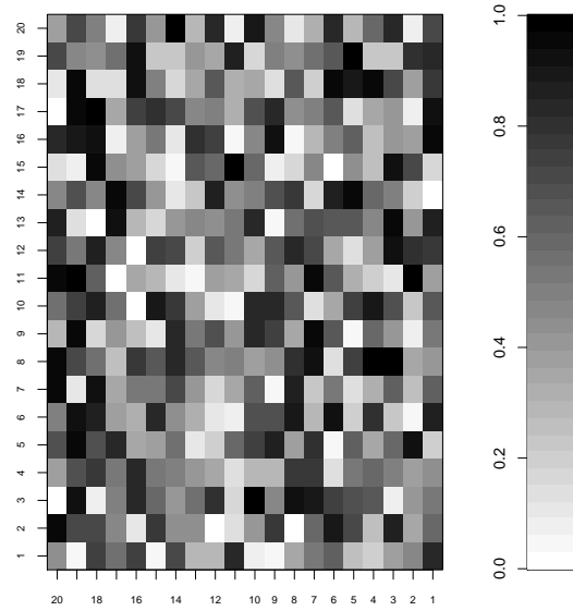
(d) A structure free transition matrix
