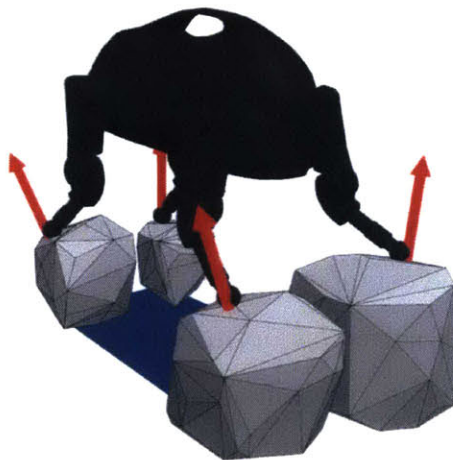
(d) Optimized posture, perspective b
