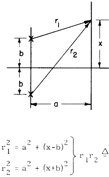
Fig. VIII-9. s-plane frequency factors.
