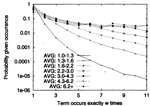
(d) Data Set 2 - Log scale
