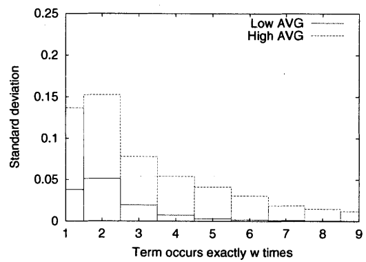
(d) avg – Data Set 2
