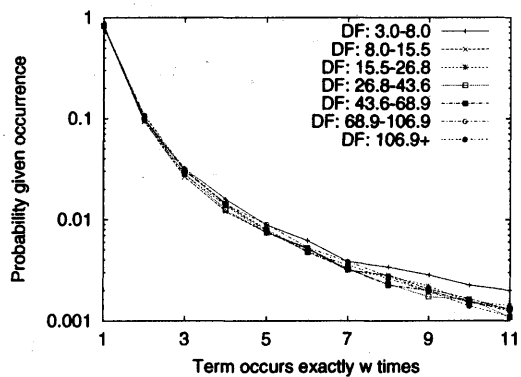
(d) Data Set 2 - Log scale
